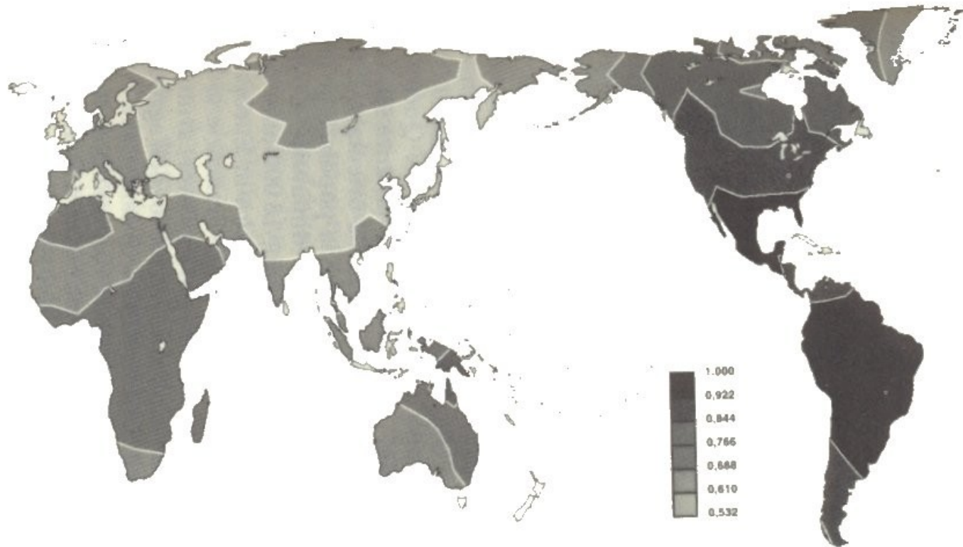
Fig. 8 Distribuzione geografica del gene 0 del sistema dei gruppi sanguigni ABO nel mondo (scala arbitraria)
